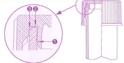
トリプルシールキャップ構造
